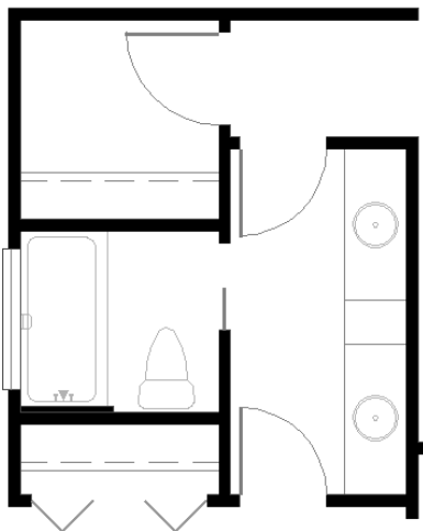
OPTIONAL JACK & JILL BATH
